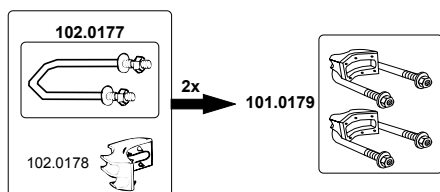
101.0179 Doppelklemme 1¼" - 2" (für z.B. 16P, 18P, 19R, 25R, 115, 500, 520, 600, 620)
